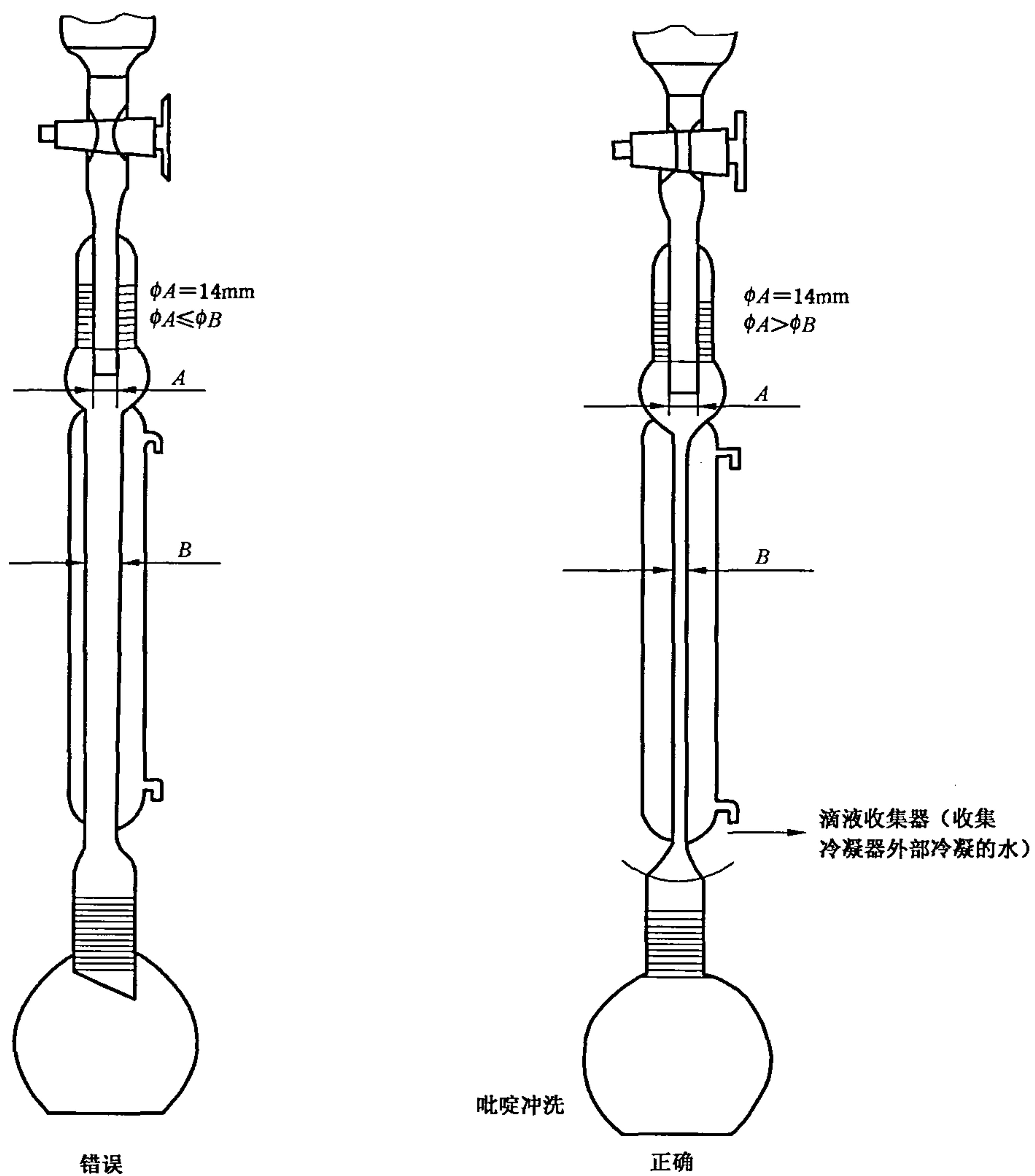
图 C.1 冷凝管实例
