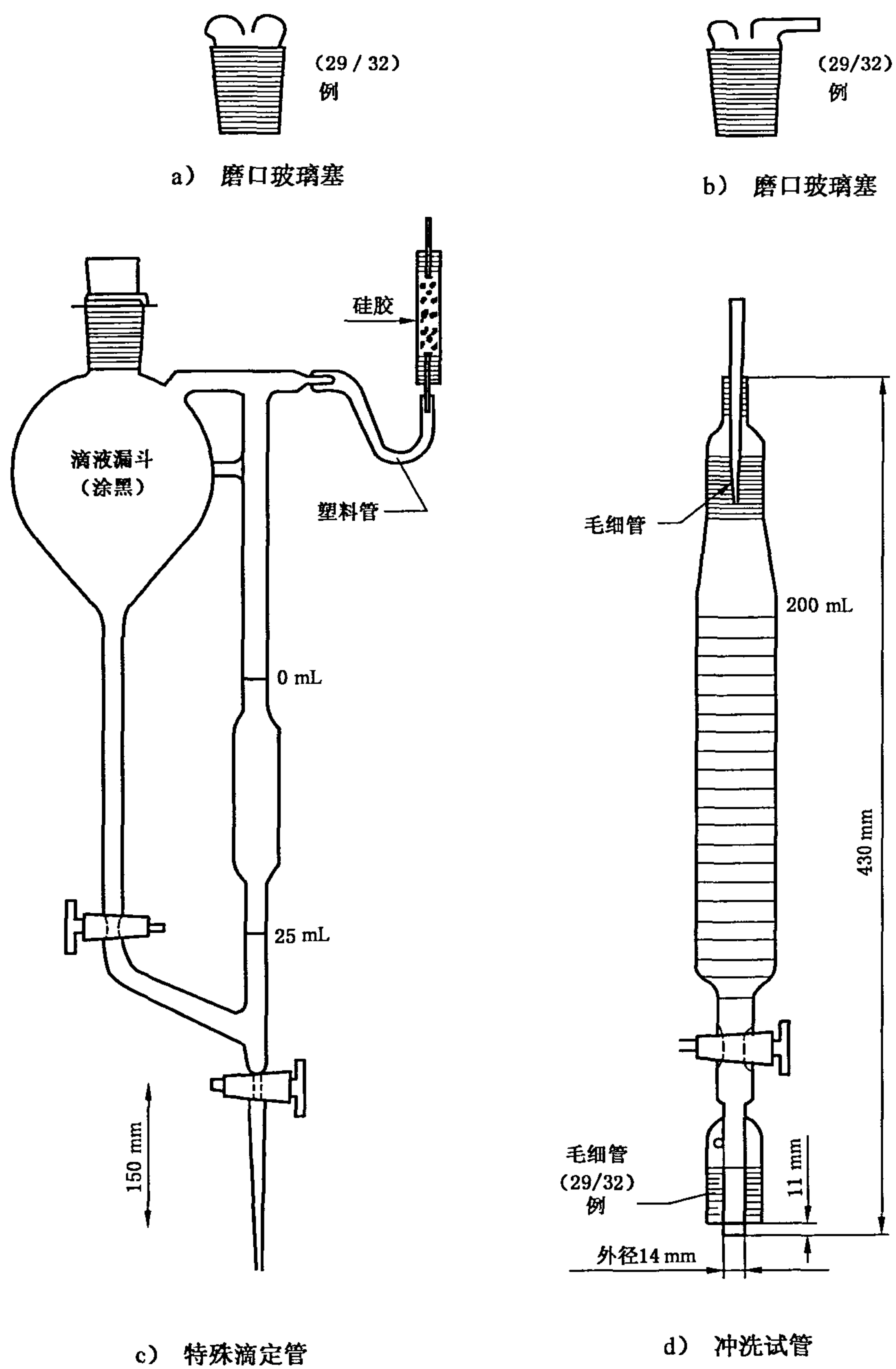
图 C.2 装置
